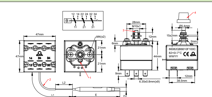
Тип с креплением при помощи центральной втулки M10
